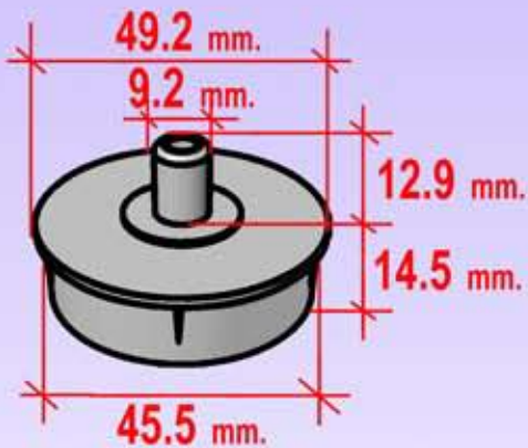
Para mandril de Ø 50 mm. Con apéndice.
